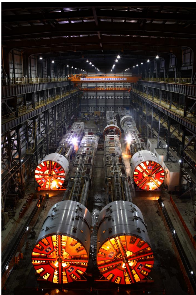
上海隧道用于新加坡地铁施工的准备出厂的盾构机
